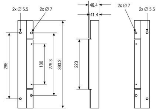
Wandhalterung für LCD-Monitore / Wall bracket for LCD monitors VMC-LCD/WMB-4
