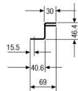
Tischstandfuß / Desktop mount
