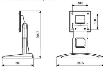
Tischstandfuß / Desktop mount
